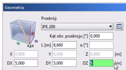
Rys. 3.44 Węzeł końcowy pręta lokalizowany przez współrzędne względne
