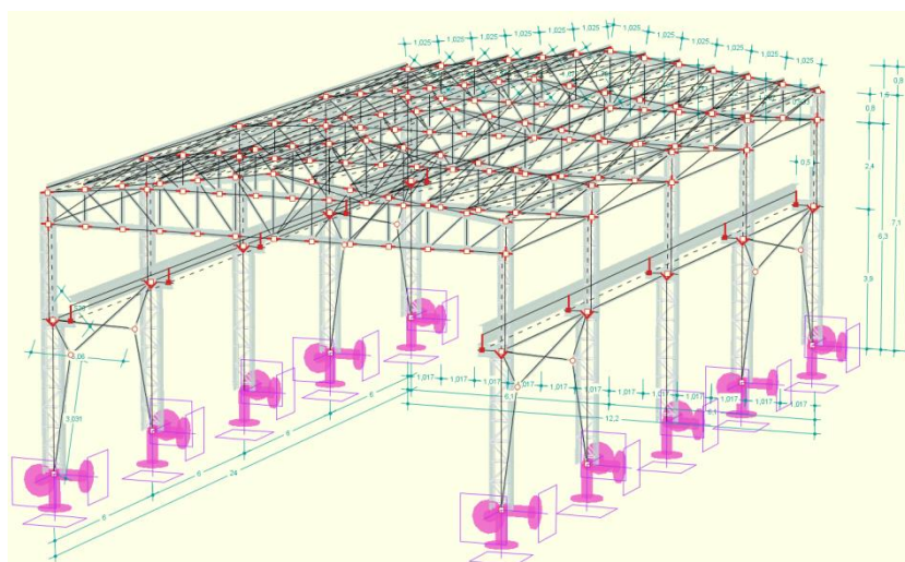
Rys. 2.7 Widok przezroczysty przekrojów prętów
