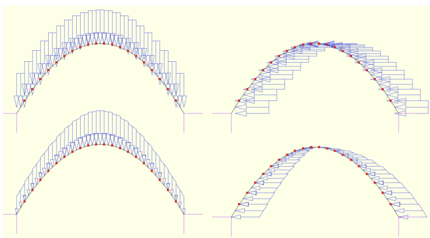
Rys. 7.16 Przykład zadanych obciążeń na rzut łuku parabolicznego (górne łuki) i odpowiadających im obciążeń prętowych (dolne łuki)
