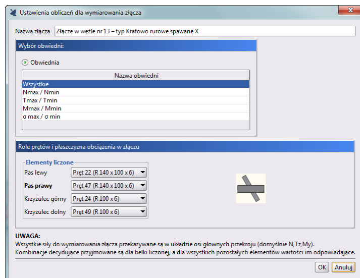
Rys. 14.46 Okno definicji złącza Kratowo rurowego spawanego typu X
