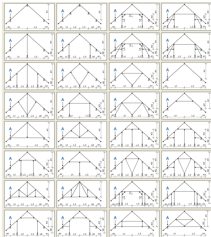
Rys. 3.52 Typy wiązarów dachowych
