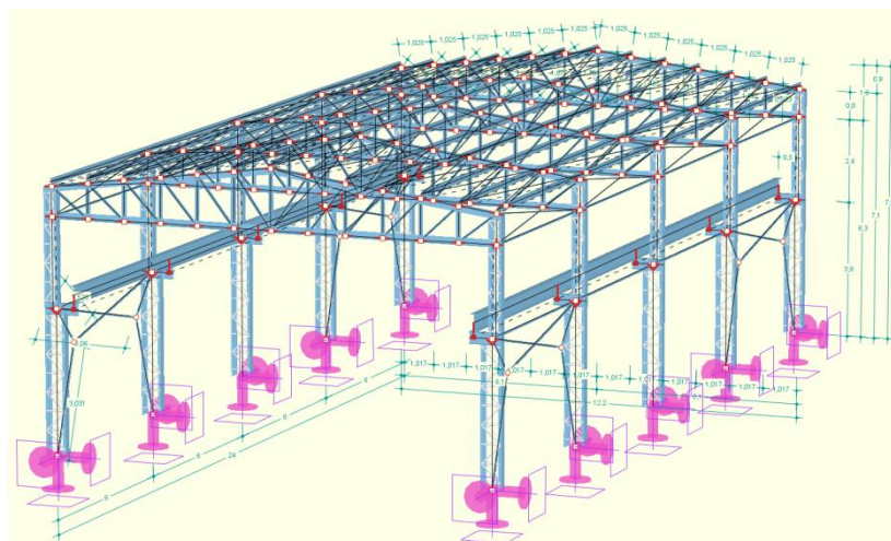
Rys. 2.6 Widok teksturowany przekrojów prętów
