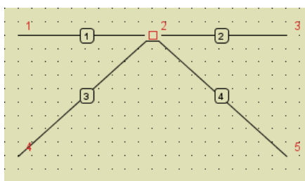
Pręty nr 3 i 4 zeszytnione, a nr 1 i 2 przegubowe
