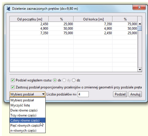
Rys. 5.16 Podział pręta względem jego rzutu
