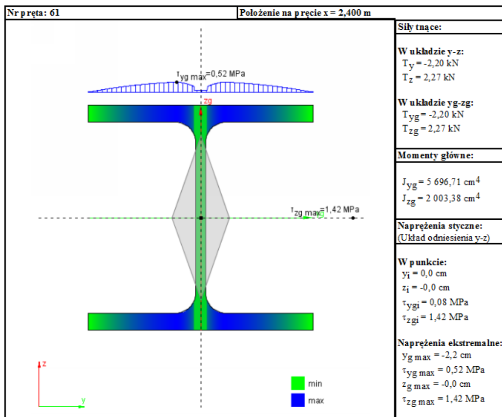
Rys. 3.74 Przykładowy raport z naprężeń stycznych w przekroju
