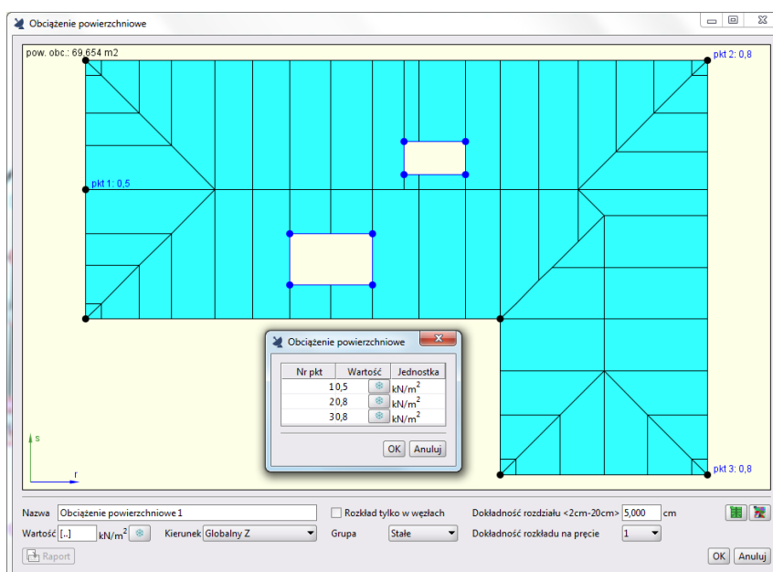
Rys. 7.39 Wpisywanie wartości obciążenia trapezowego w zdefiniowanych punktach
