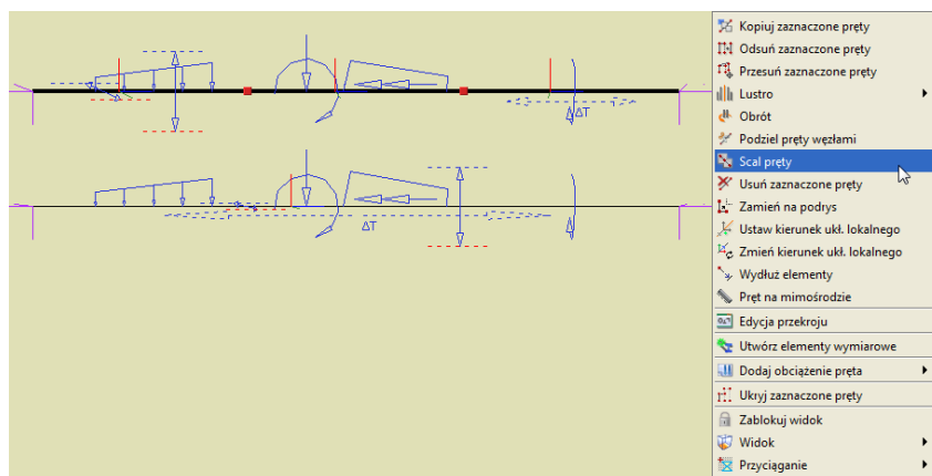
Rys. 5.20 Wywołanie funkcji scalania i widok obciążeń przed i po scaleniu
