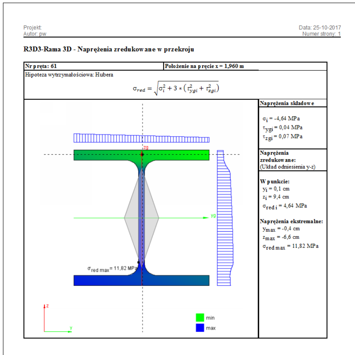
Rys. 3.76 Przykładowy raport z naprężeń zredukowanych w przekroju
