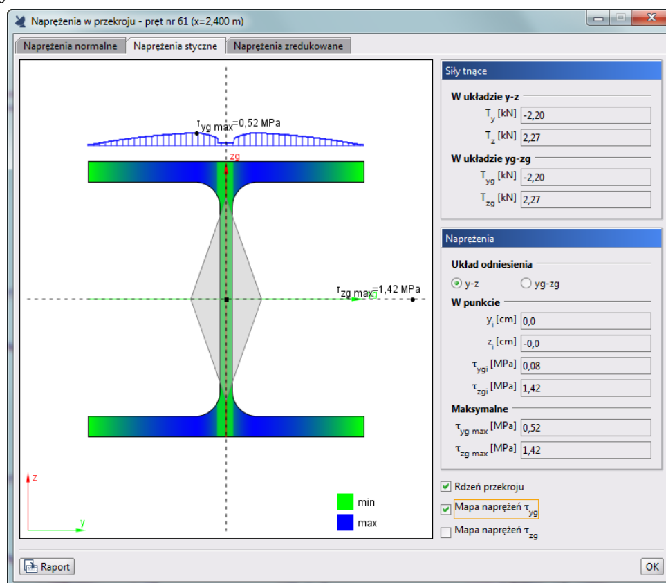
Rys. 3.73 Napężenia styczne w przekroju
