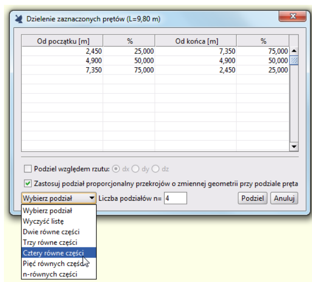
Rys. 5.14 Podział prętów węzłami
