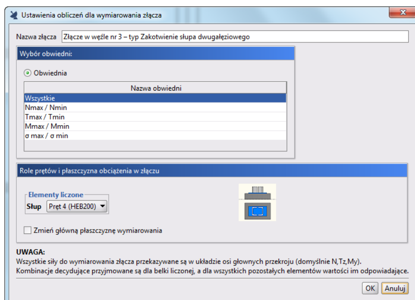
Rys. 14.50 Okno definicji zakotwienia słupa dwugąłżowego
