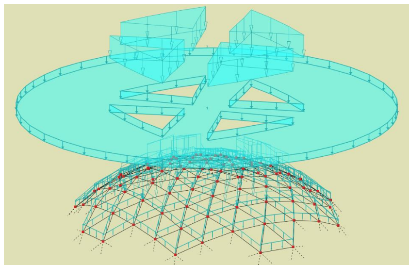
Rys. 7.42 Przykłady wykorzystania otworów zdefiniowanych w obszarze obciążenia powierzchniowego
