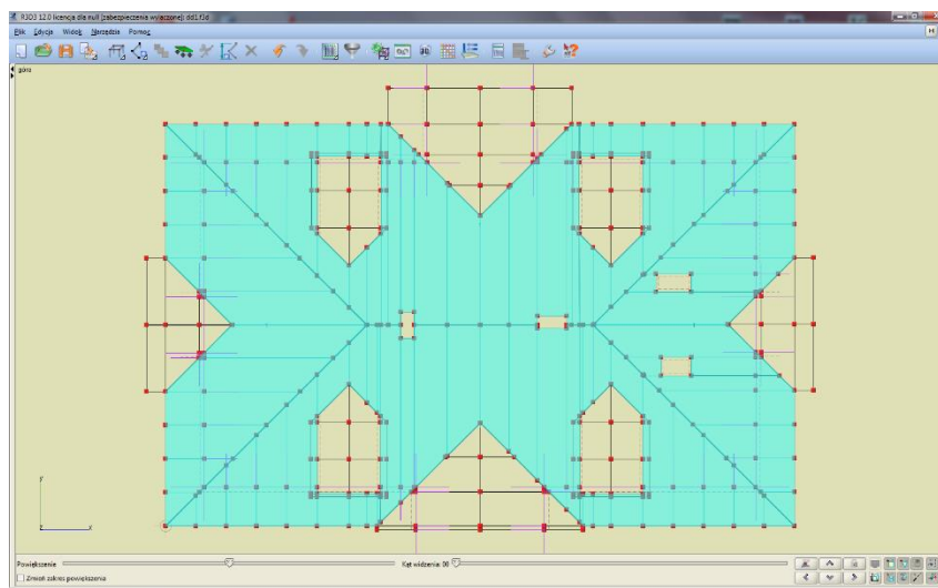
Rys. 7.36 Przykład modelowania obciążenia powierzchniowego (pionowego od ciężaru pokrycia) na głównych połaciach, z uwzględnieniem otworów w połaci
