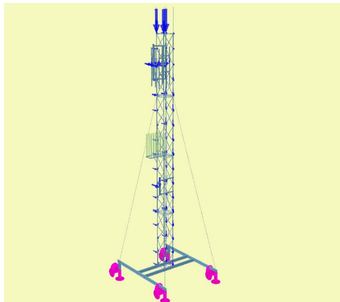
Rys. 13.7 Maszt telekomunikacyjny
