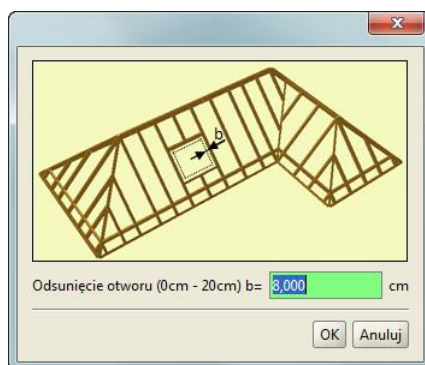
Rys. 2.45 Okno edycji odsunięcia osi elementów konstrukcji od krawędzi otworu połaciowego dla danego otworu
