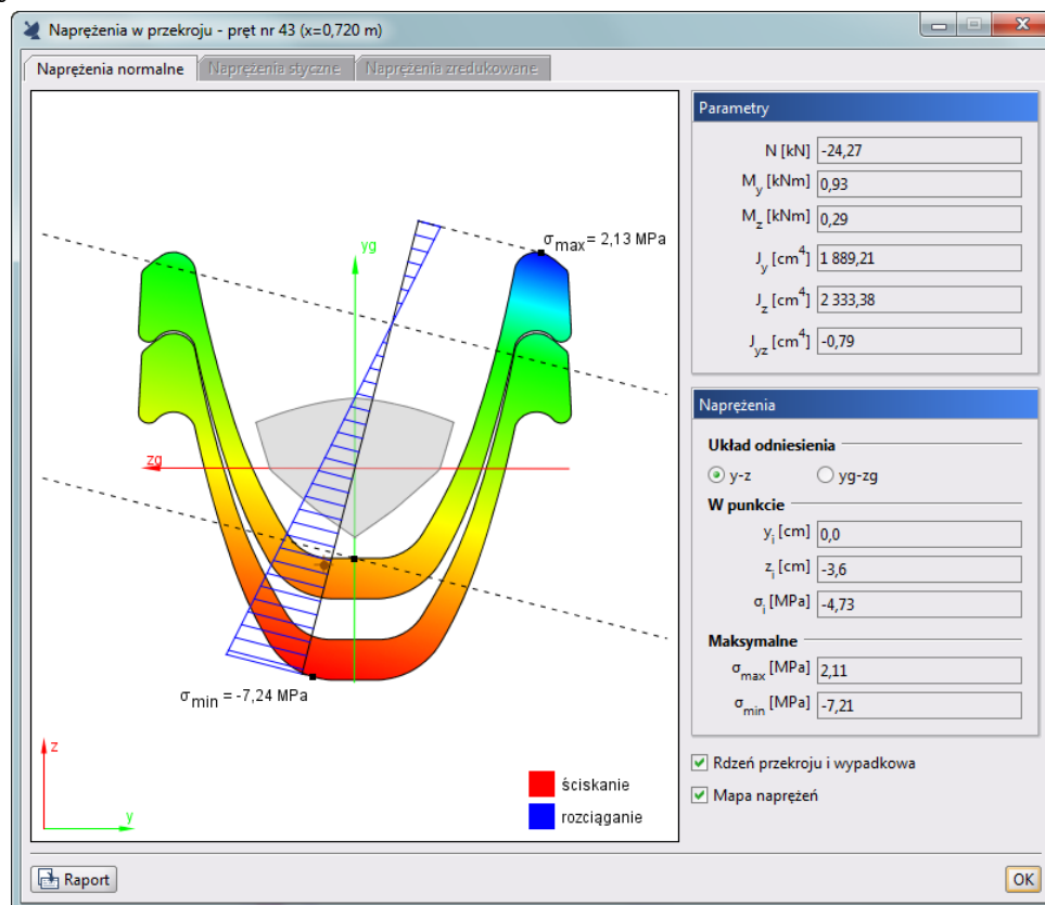
Rys. 3.70 Napężenia w przekroju
