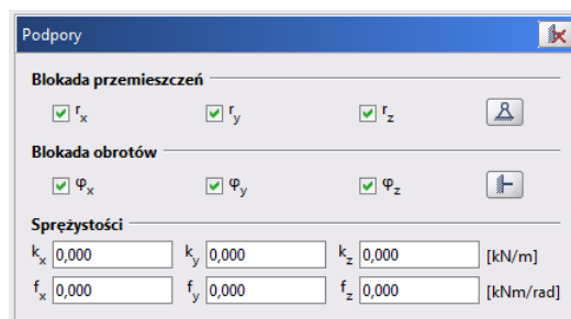
Rys. 6.3 Podpory
