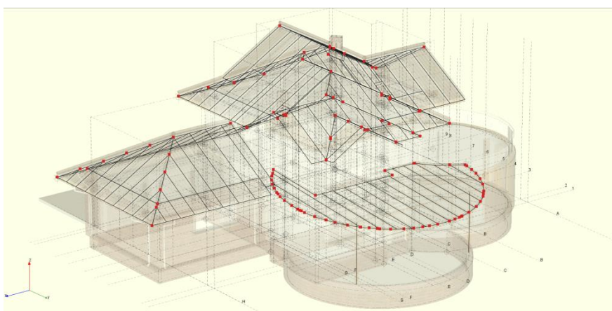
Rys. 2.12 Widok przezroczystego modelu z ArCADii
