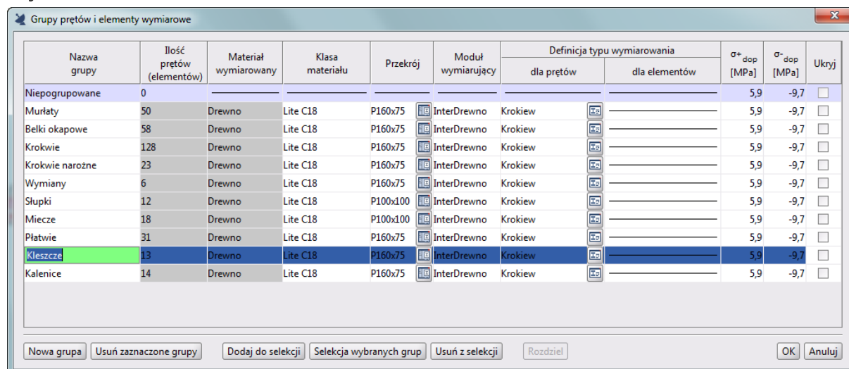
Rys. 14.7 Okno edycji grup prętów i elementów wymiarowych
