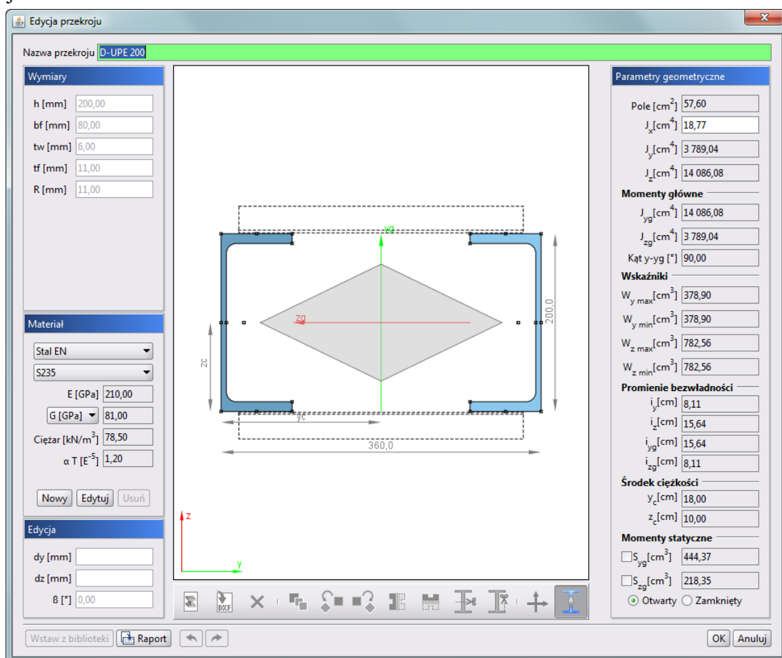
Rys. 4.20 Okno Edytora przekroju dla profili złożonych
