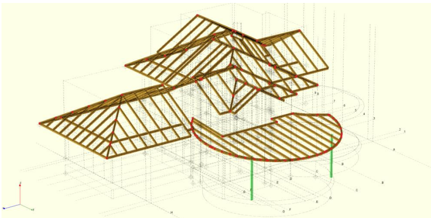
Rys. 2.13 Widok wyłączanego modelu z ArCADii z renderowanym widokiem prętów i włączonym wyświetlaniem podrysów
