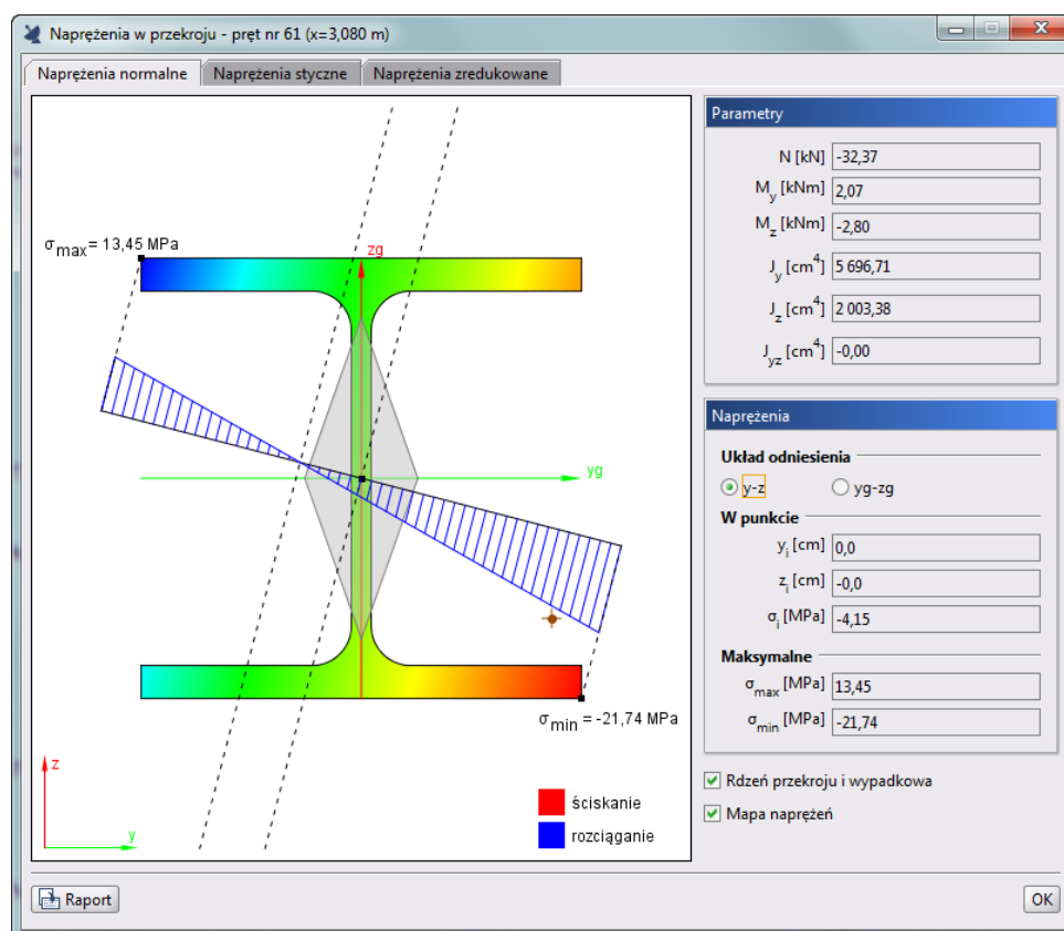
Rys. 3.71 Naprężenia normalne w przekroju
