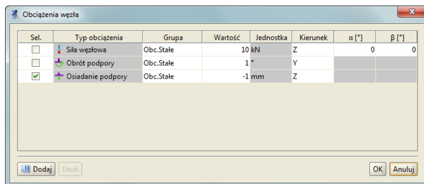
Rys. 3.55 Obciążenia pręta, węzła i podpory
