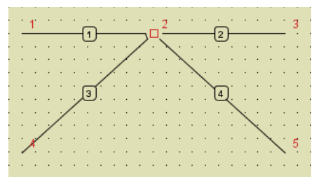
Pręty nr 1 i 3 zeszytnione, a nr 2 i 4 przegubowe
