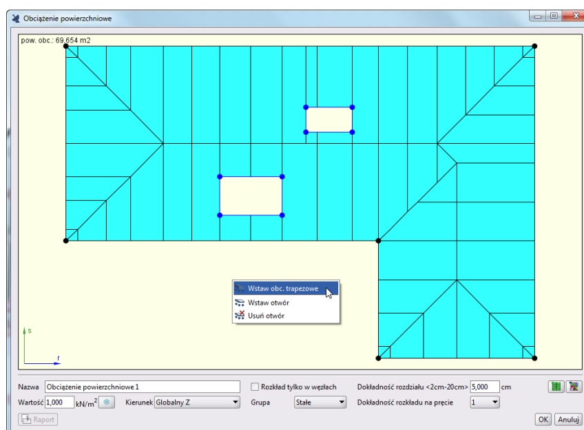
Rys. 7.38 Definiowanie obciążenia trapezowego
