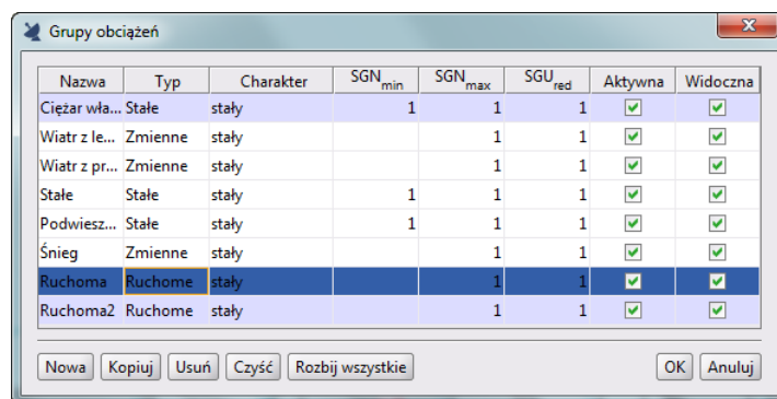
Rys. 7.24 Grupa obciążenia ruchomego
