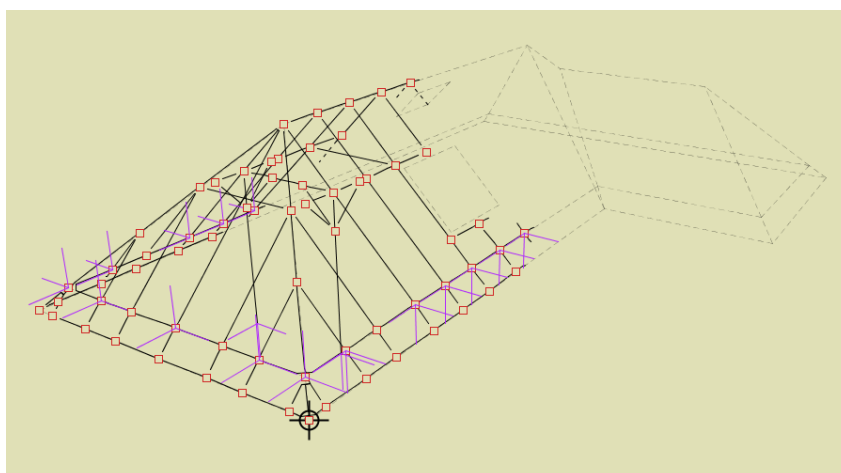
Rys. 2.28 Widok przestrzennego podrysu z częściowo wprowadzonym układem
