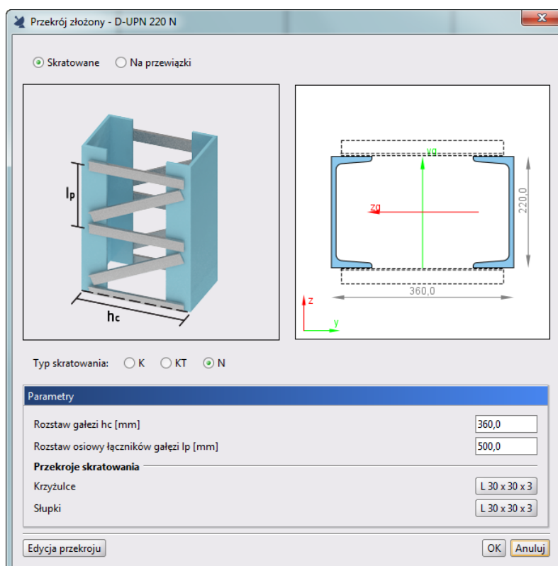
Rys. 4.18 Okno pośrednie dla profili złożonych dalekogałęziowych (dwugałęziowych)
