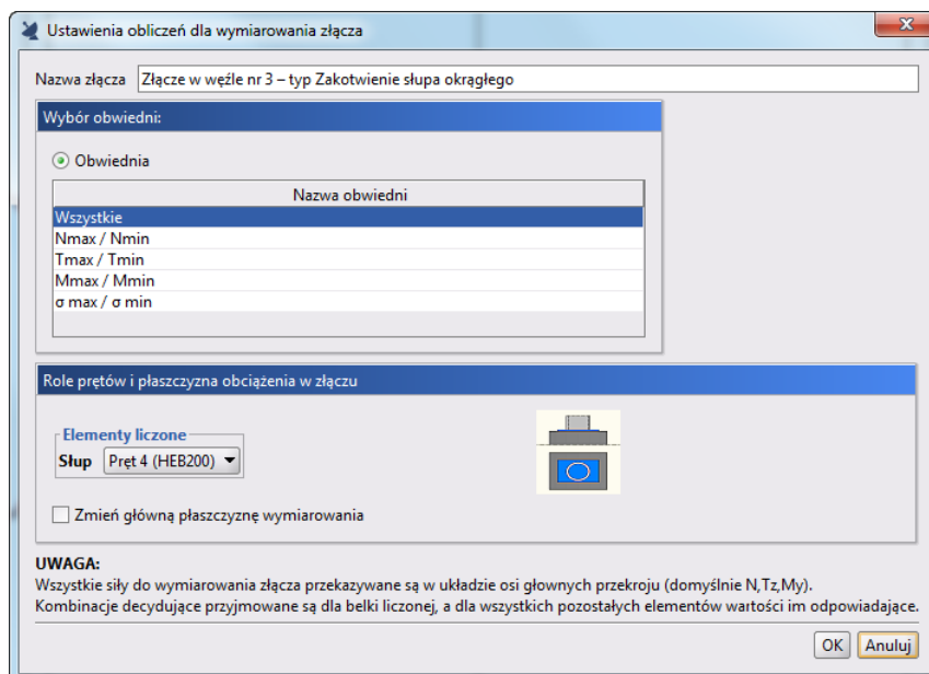
Rys. 14.53 Okno definicji zakotwienia słupa okrągłego
