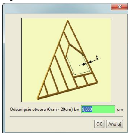
Rys. 2.46 Okno edycji odsunięcia osi elementów konstrukcji od krawędzi otworu facjatki dla danego otworu facjatki
