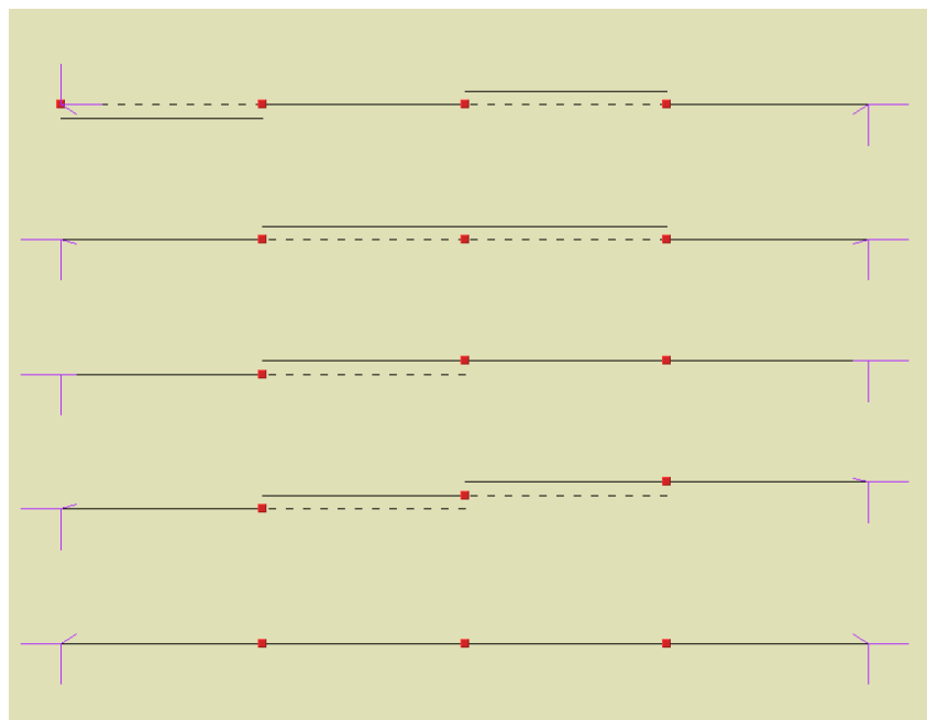
Rys. 7.21 Układy prętów z mimośrodkami, na których można wprowadzić obciążenie ruchome
