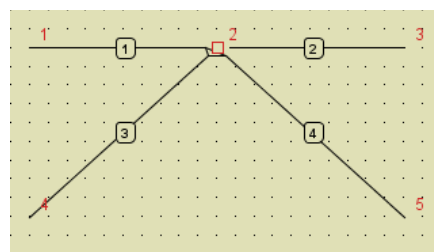
Pręty nr 1, 3 i 4 zeszytnione, a nr 2 przegubowy
