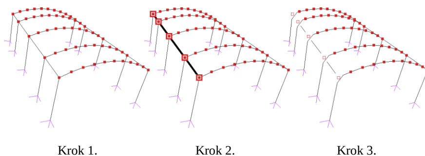
Rys. 5.10 Wprowadzanie przegubów w płatwiach
