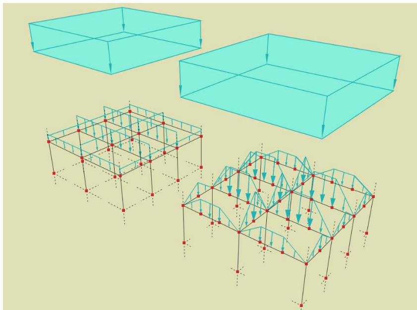
Rys. 7.43 Dwa różne rozkłady takiego samego obciążenia zależnie od podziału prętów
