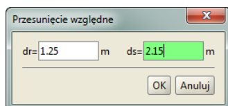
Rys. 7. 35 Przesunięcie względne punktu na konturze obszaru obciążenia
