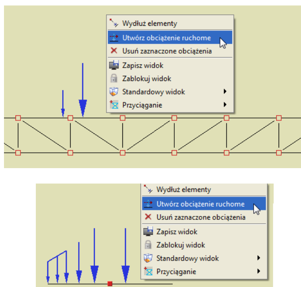
Rys. 7.17 Przykłady „zespołu pojazdu”, z których można utworzyć obciążenie ruchome
