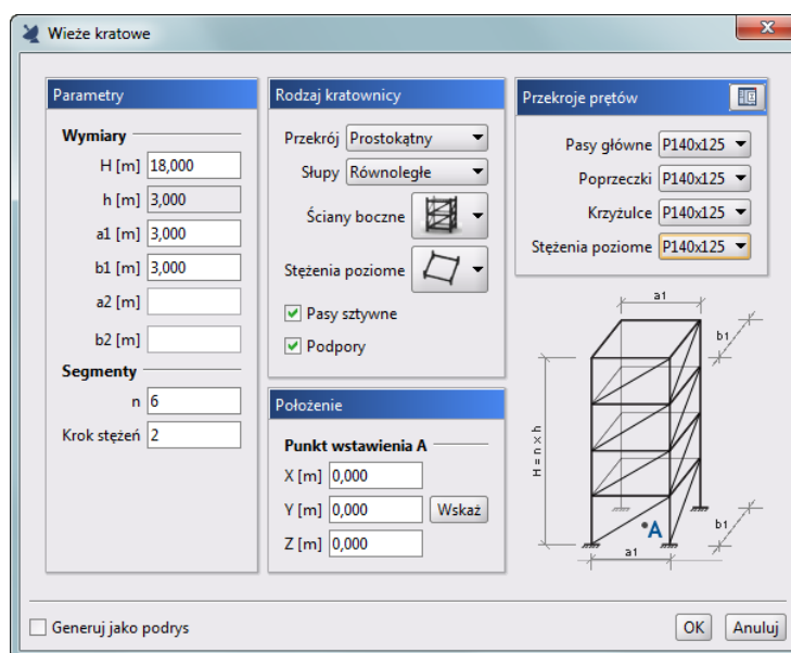
Rys. 3.53 Wieże kratowe
