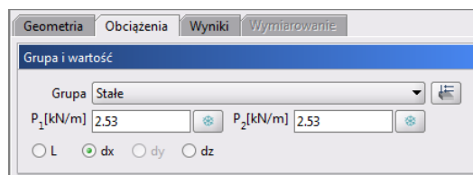
Rys. 7.13 Znaczniki obciążeń zadawanych na rzut pręta na zakładce Obciążenia
