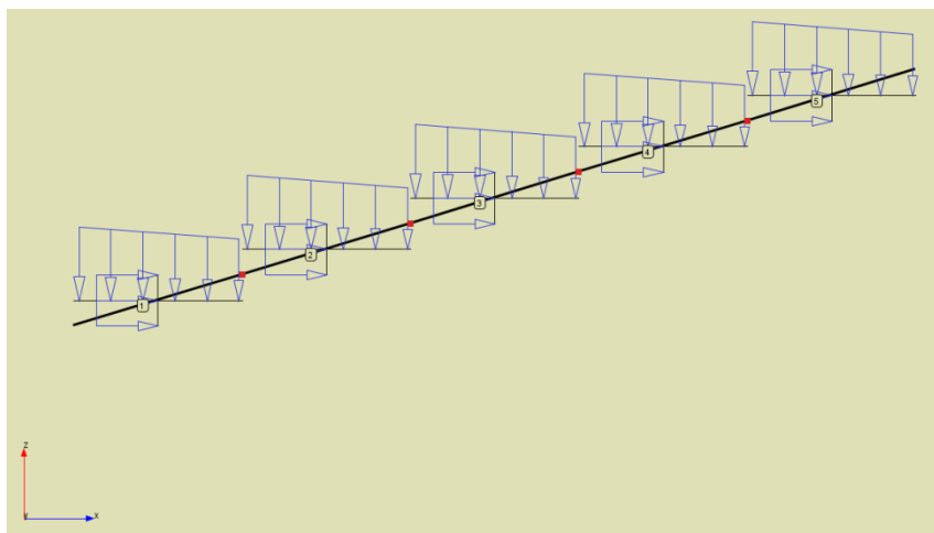
Rys. 7.14 Reprezentacja graficzna obciążeń zadanych na rzut prętów
