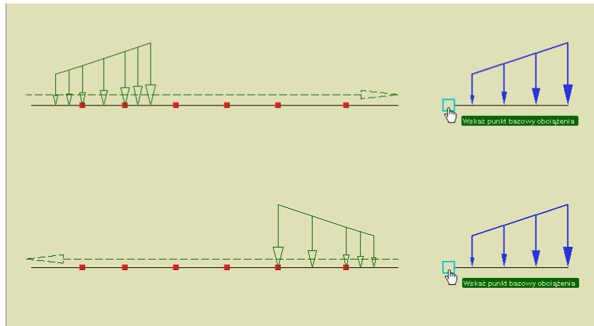
Rys. 7.20 Przykład obciążenia wyjściowego i jego widok na wektorze przemieszczenia
