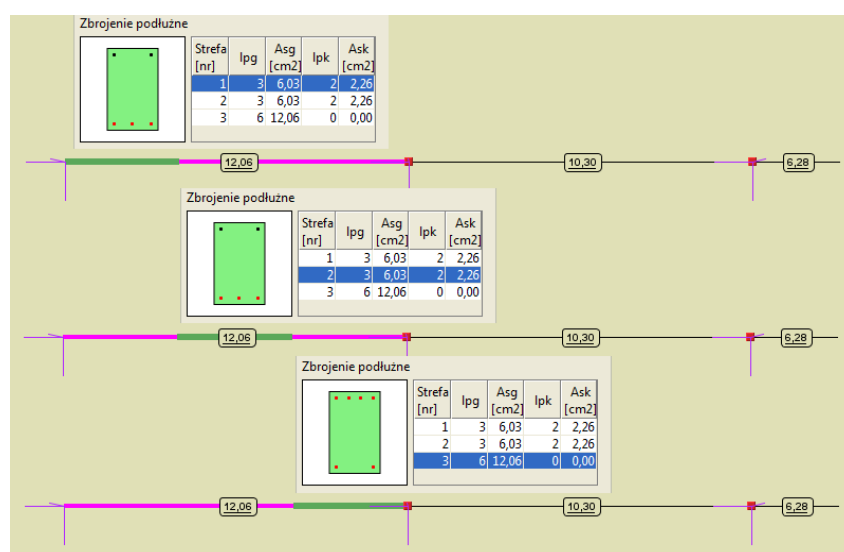
Rys. 14.18 Widok stref zbrojenia belki
