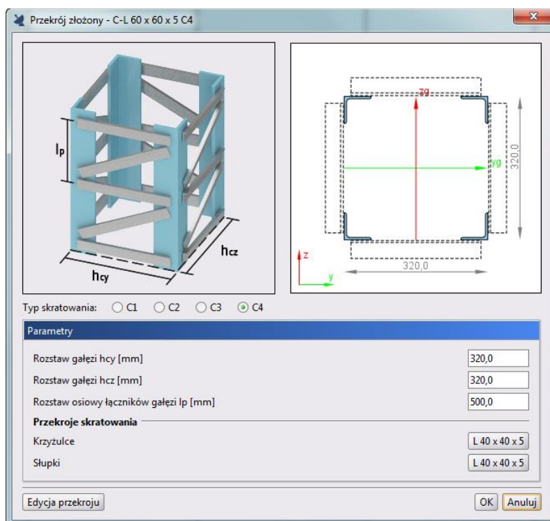
Rys. 4.19 Okno pośrednie dla profili złożonych dalekogałęziowych (czterogałęziowych)
