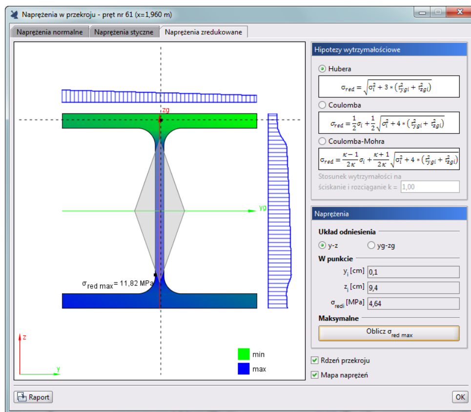
Rys. 3.75 Naprężenia zredukowane w przekroju
