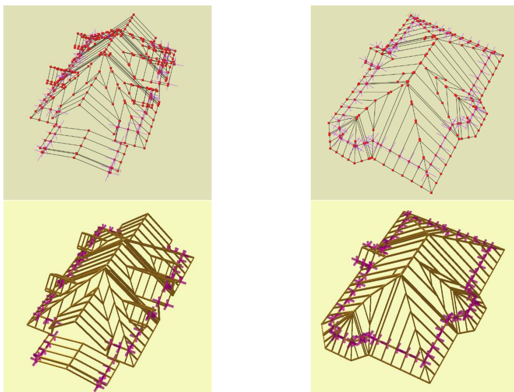
Rys. 2.42 Przykłady projektów dachów z systemu ArCADia z automatycznie wygenerowanym układem konstrukcji połaci w modelu siatkowym i widoku 3D
