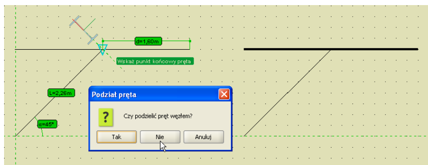
Rys. 3.87 Wprowadzany pręt niepołączony (luźny)
