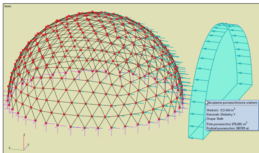
Rys. 7.48 Przykłady zadanych obciążeń powierzchniowych
