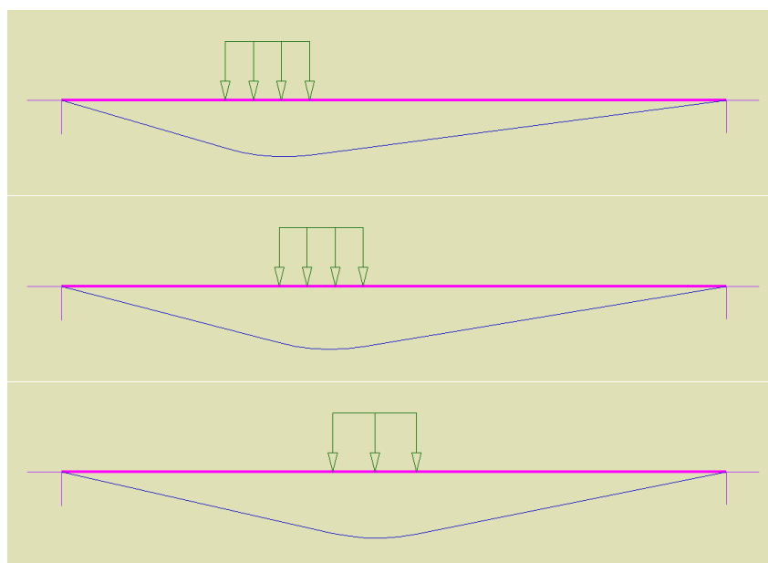
Rys. 7.31 Widoki przemieszczającego się obciążenia ruchomego
