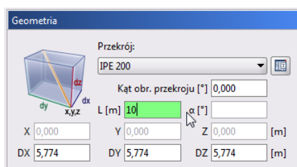
Rys. 3.45 Węzeł końcowy pręta lokalizowany przez podanie długości pręta we wskazanym kierunku
