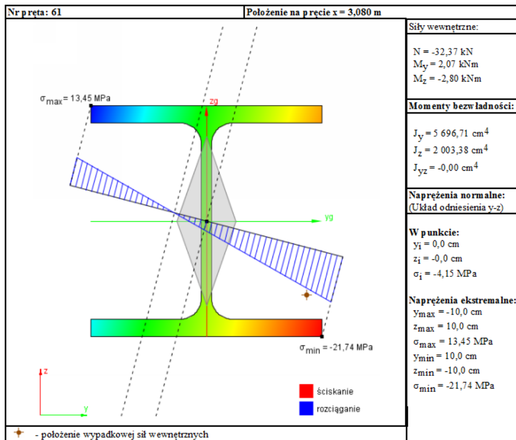
Rys. 3.72 Przykładowy raport dla naprężeń normalnych
