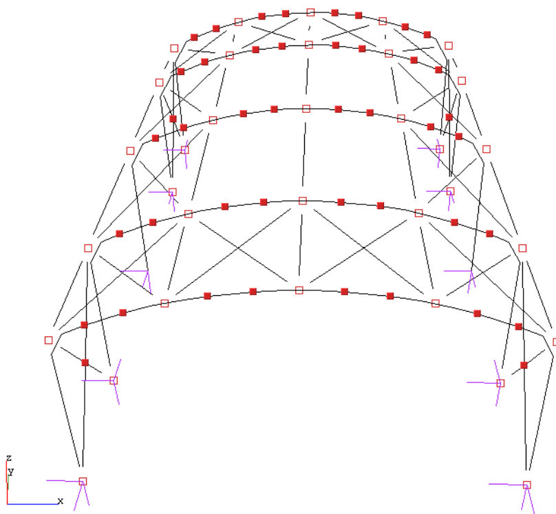
Rys. 5.1 Przykładowa konstrukcja
