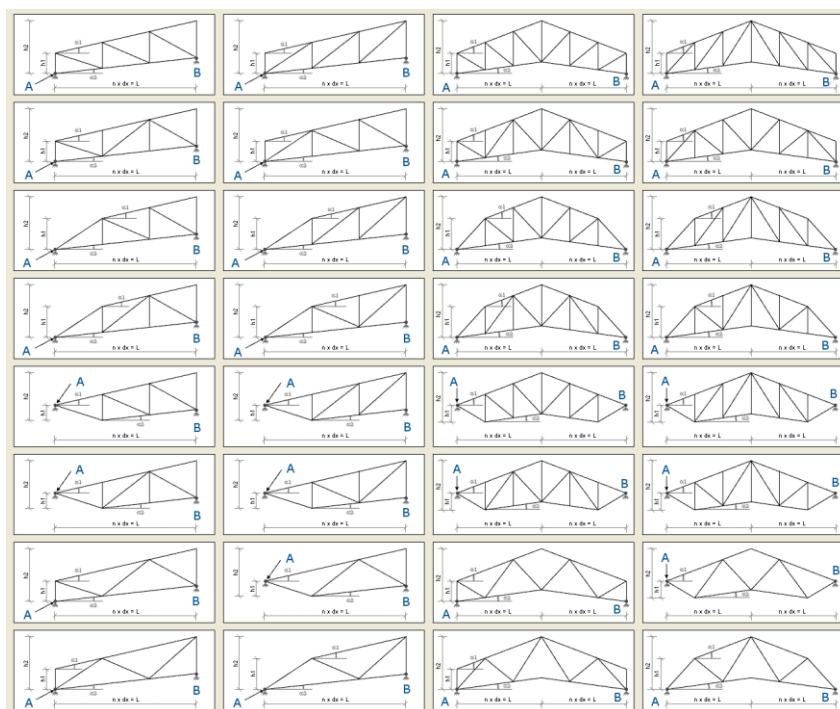
Rys. 3.50 Typy kratownic płaskich
