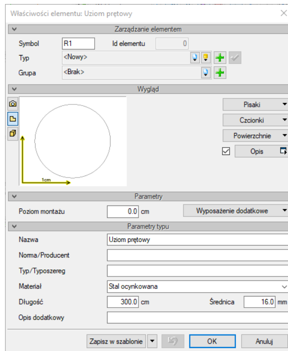
Rys. 32 Okno właściwości uziomu prętowego
