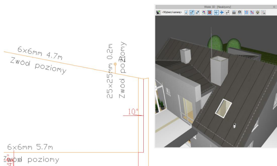
Rys. 22 Iglica aktywna w przykładowym projekcie
