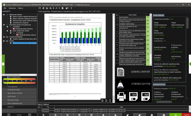
Rysunek 16. ARCADIA-TERMOCAD PCHE - efekt ekonomiczny
