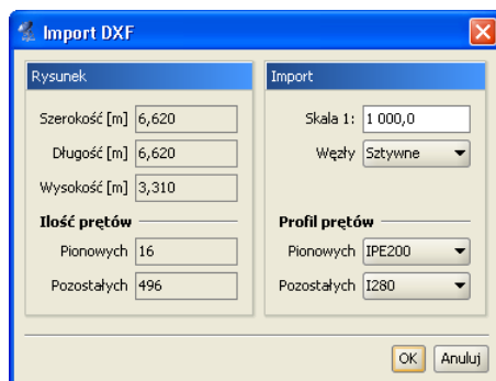
Rys. 2.9 Okno importu rysunków DXF
