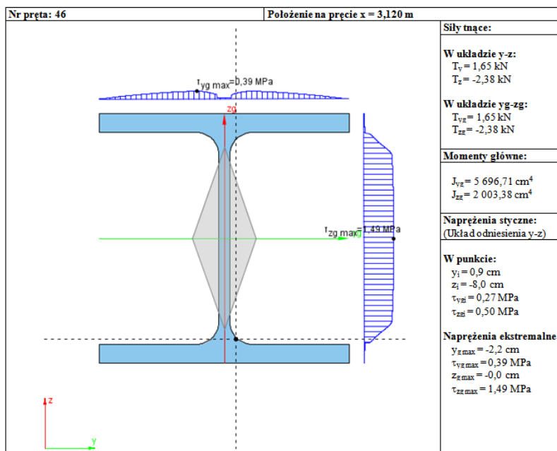
Rys. 3.45 Przykładowy raport z naprężeń stycznych w przekroju
