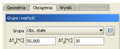
Rys. 7.8 Różnica temperatur
