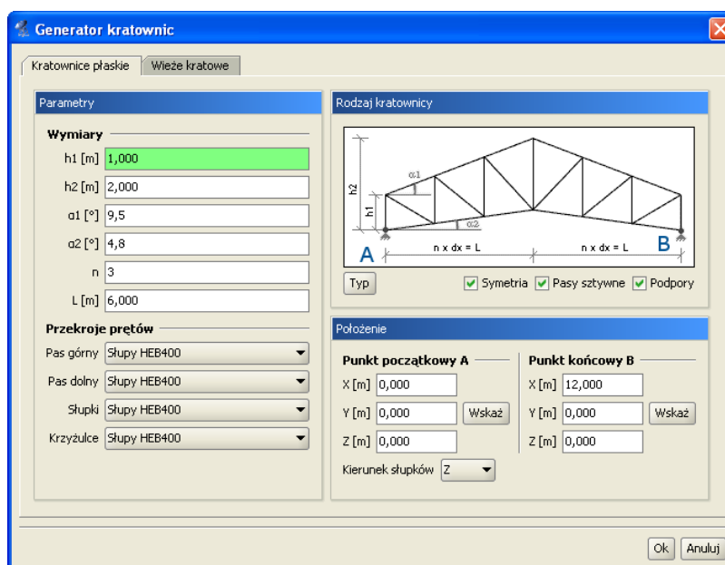
Rys. 3.32 Generator kratownic płaskich
