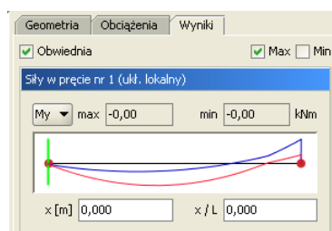
Rys. 11.5 Wykresy obwiedni dla pojedynczego pręta
