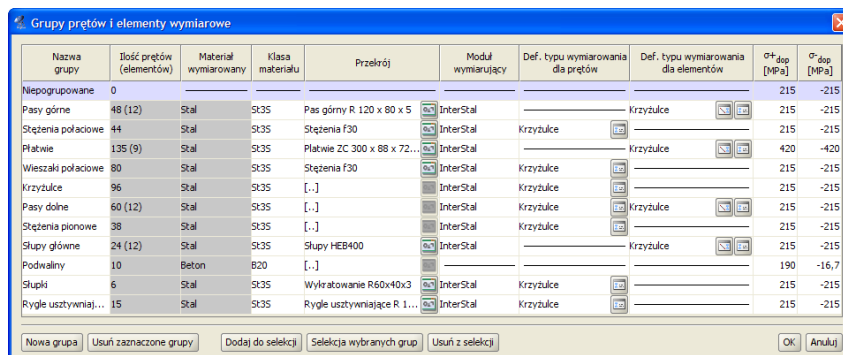
Rys. 14.7 Okno edycji grup prętów i elementów wymiarowych
