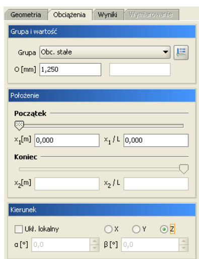
Rys. 7.9 Osiadanie podpory
