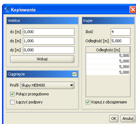
Rys. 3.37 Kopiowanie
