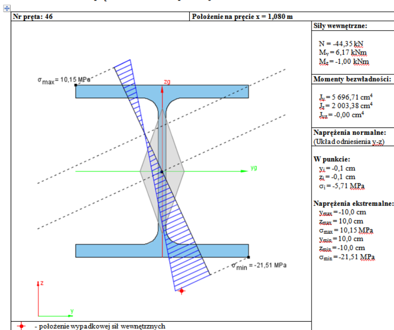
Rys. 3.43 Przykładowy raport dla naprężeń normalnych
