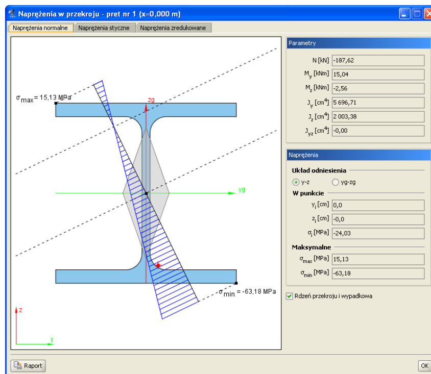
Rys. 3.41 Naprężenia w przekroju
