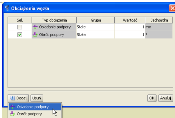
Rys. 6.7 Okna edycji obciążeń prętowych i podporowych dla pojedynczego pręta lub węzła podporowego
