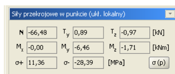
Rys. 11.6 Siły przekrojowe w punkcie
