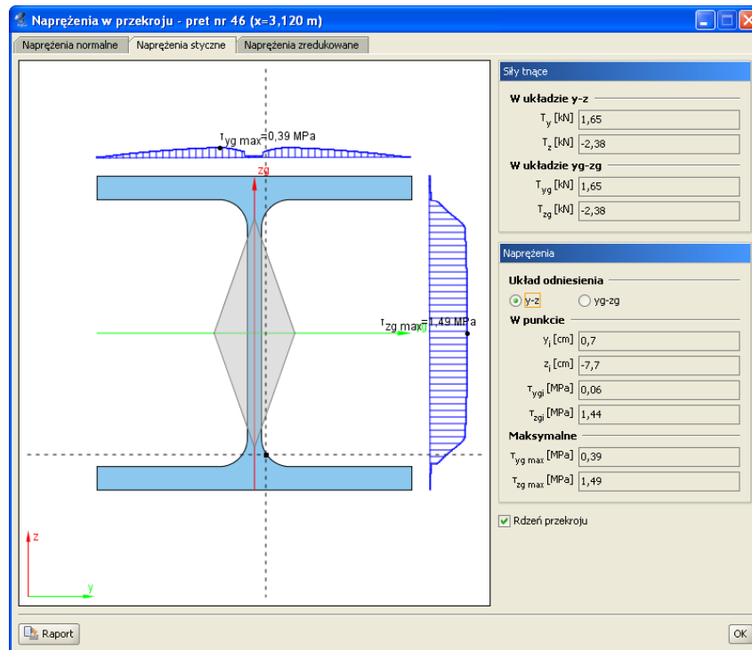
Rys. 3.44 Napężenia styczne w przekroju
