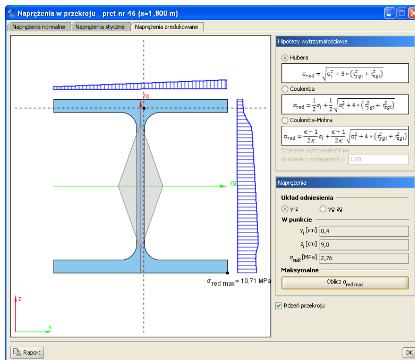
Rys. 3.46 Naprężenia zredukowane w przekroju
