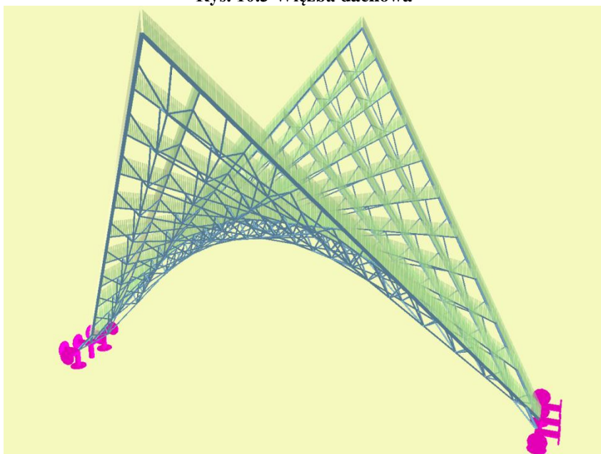
Rys. 10.4 Przekrycie strukturalne - prostokreślne
