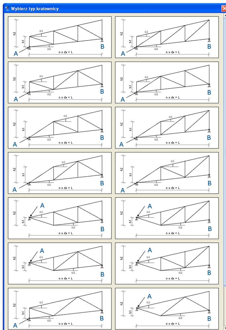
Rys. 3.33 Typy kratownic płaskich
