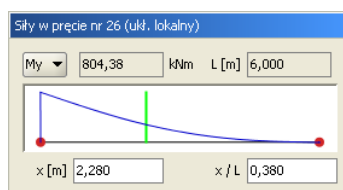
Rys. 11.3 Wykresy sił dla pojedynczego pręta
