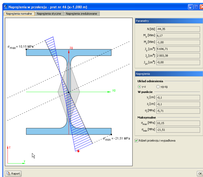
Rys. 3.42 Naprężenia normalne w przekroju
