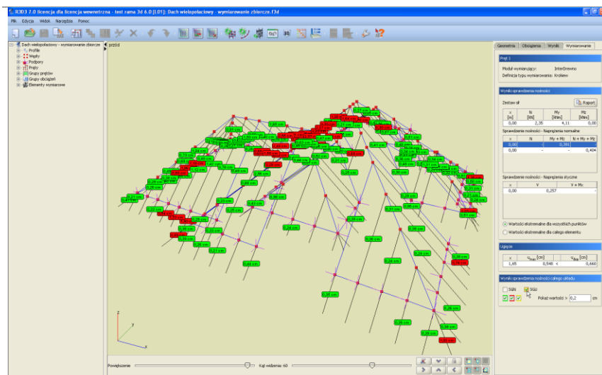
Rys. 14.19 Widok wyników wymiarowania zbiorczego dla stanu granicznego użytkowania
