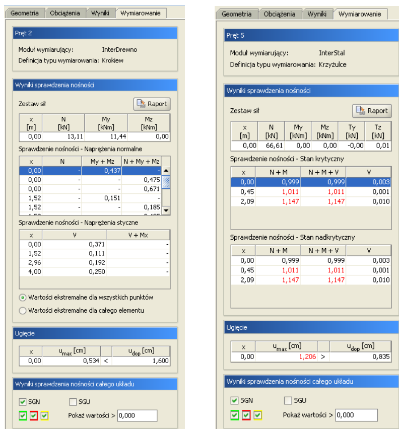
Rys. 14.13 Widok zakładek Wymiarowanie dla elementu drewnianego i stalowego
