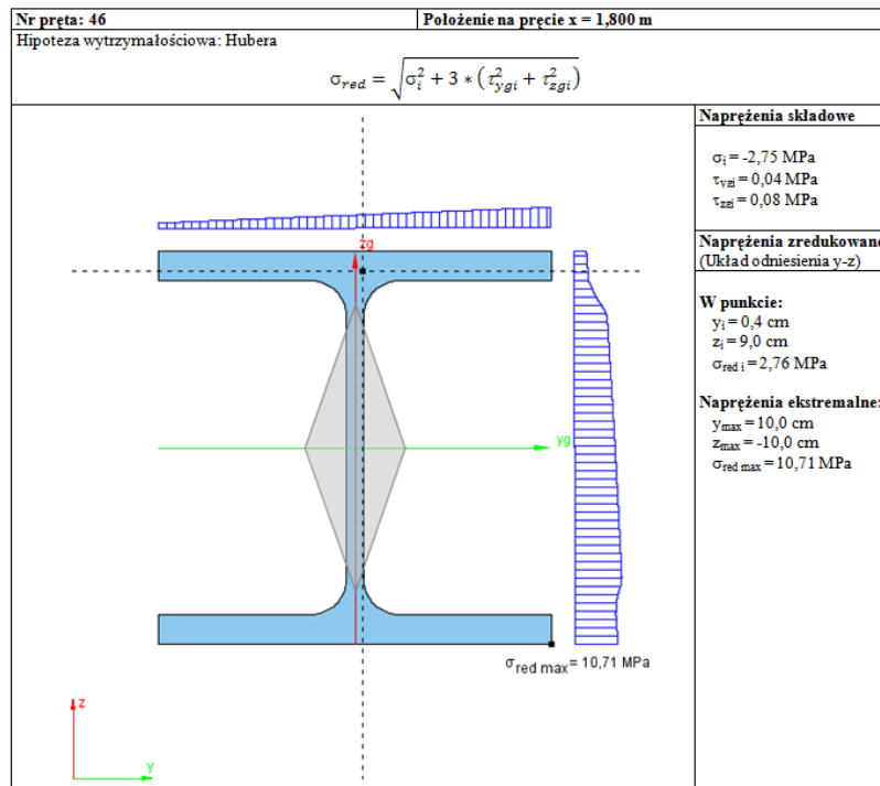
Rys. 3.47 Przykładowy raport z naprężeń zredukowanych w przekroju
