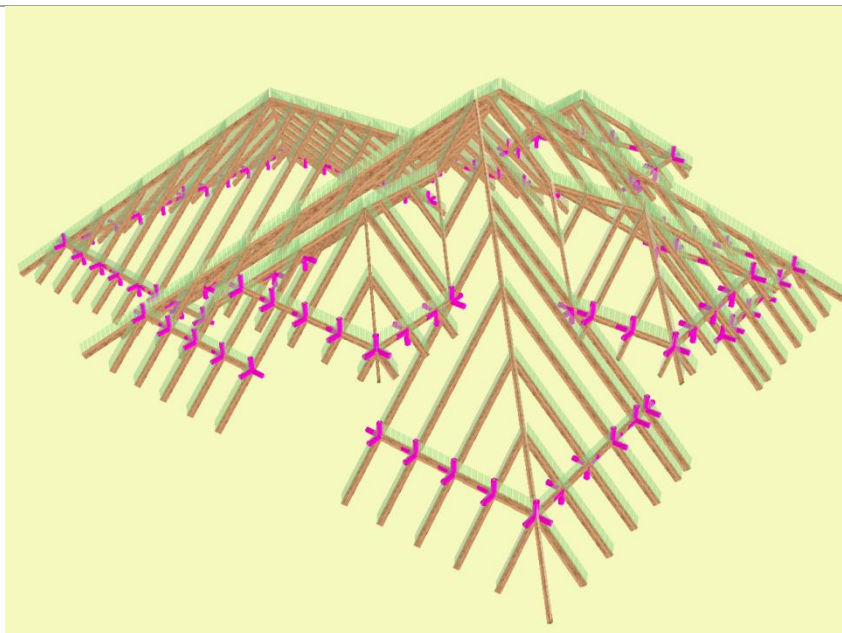
Rys. 10.3 Wieżba dachowa
