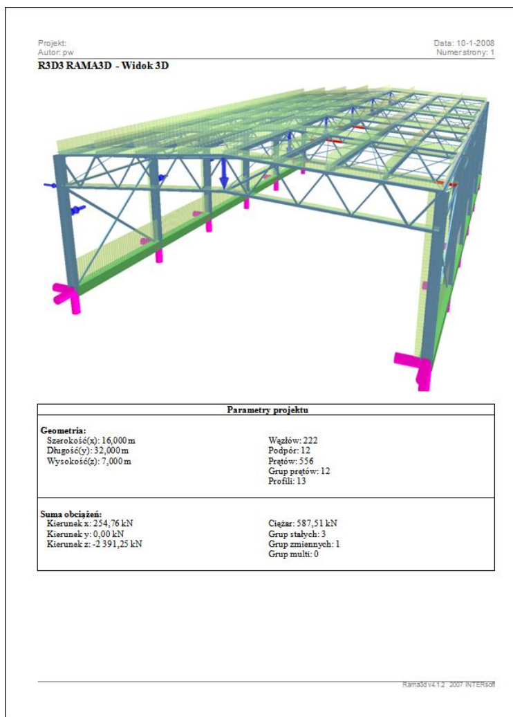
Rys. 3.15 Raport z Widoku 3D
