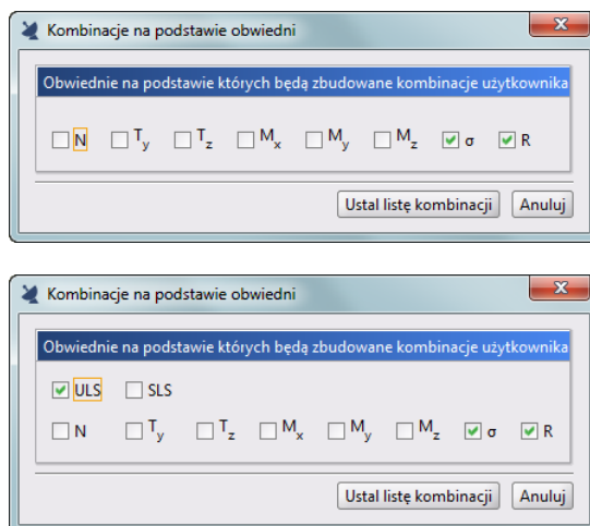
Okna ustawień Kombinacji na podstawie obwiedni dla projektów PN i PN-EN
