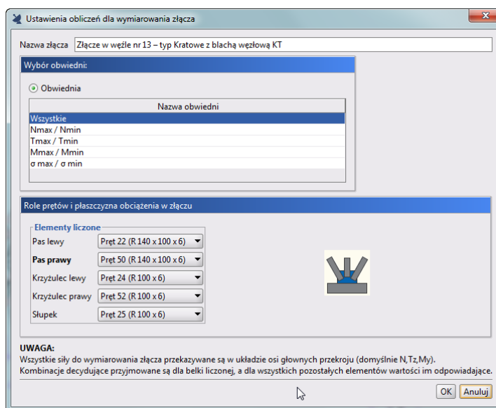
Okno definicji złącza Kratowego z blachą węzłową typu KT
