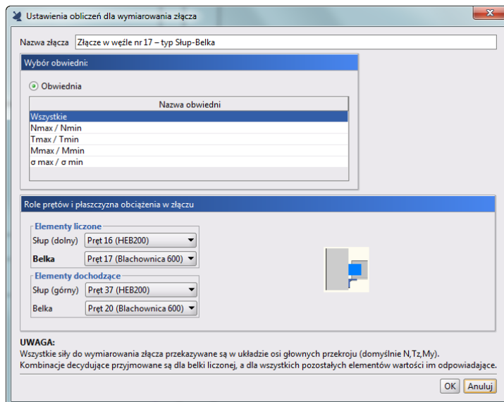
Okno definicji złącza Stup-Belka
