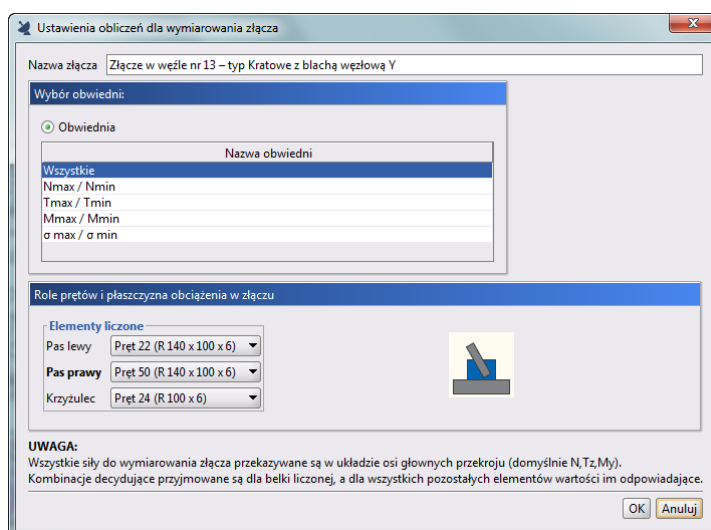
Okno definicji złącza Kratowego z blachą węzłową typu Y
