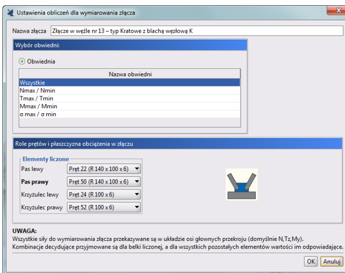
Okno definicji złącza Kratowego z blachą węzłową typu K
