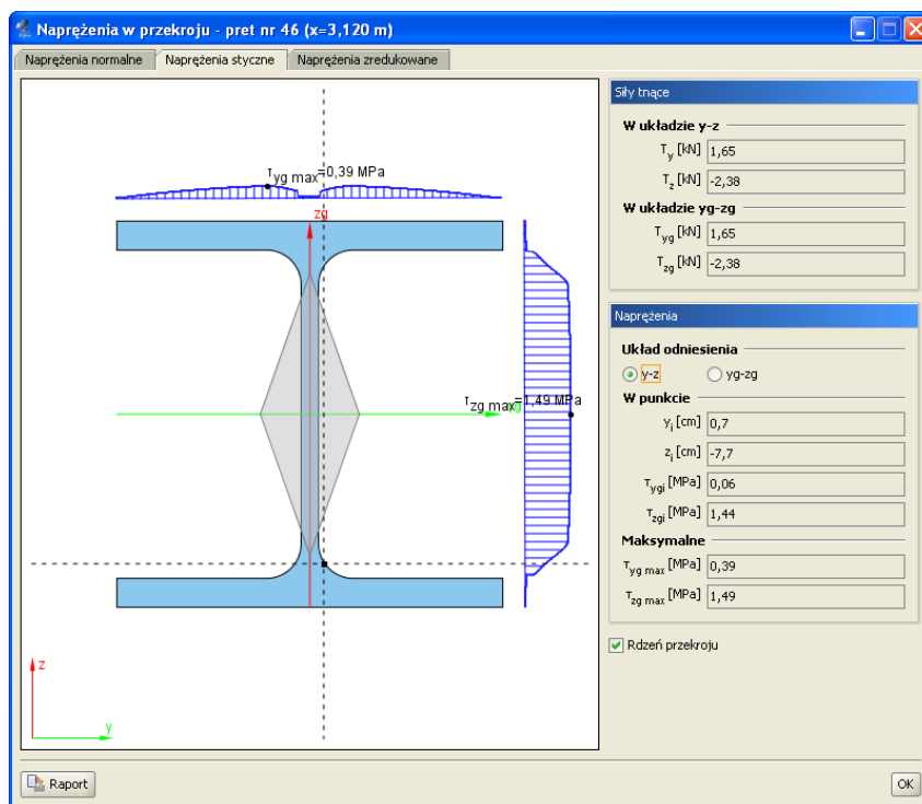
Rys. 3.68 Napężenia styczne w przekroju
