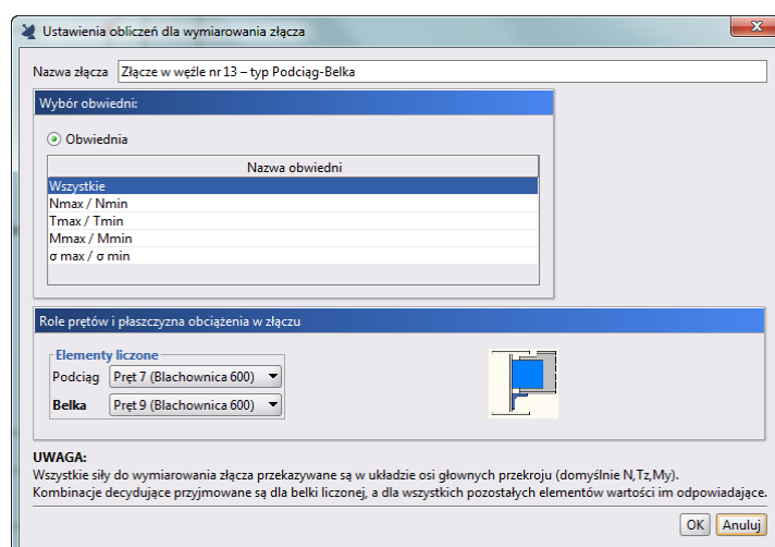
Okno definicji złącza Podciąg-Belka
