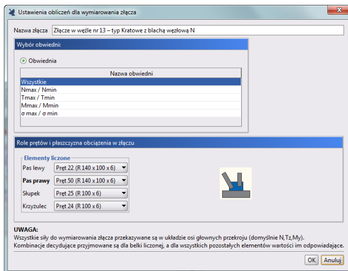
Okno definicji złącza Kratowego z blachą węzłową typu N
