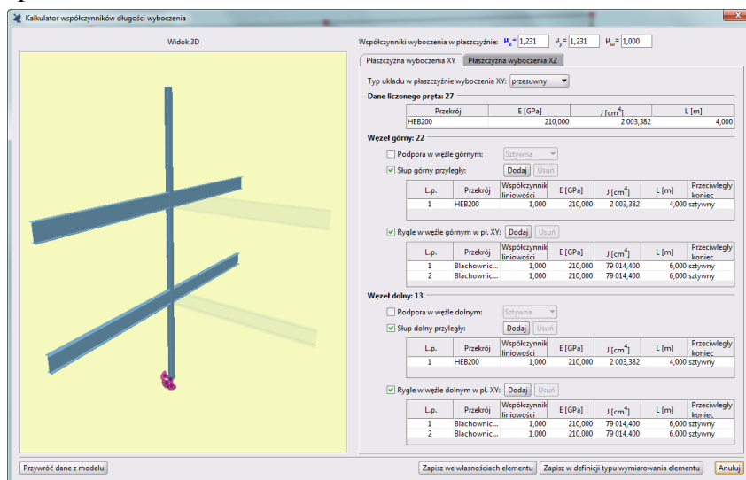
Widok okna kalkulatora po przywróceniu danych z modelu
