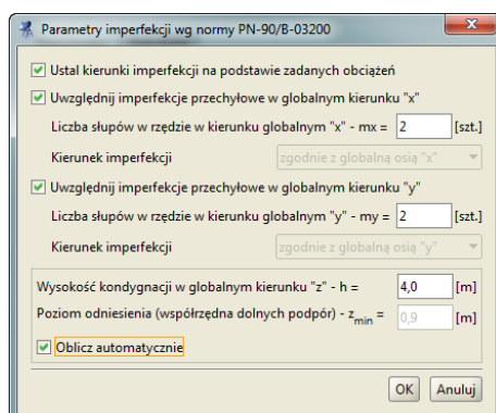
Rys. 10.4 Okno Parametrów imperfekcji dla PN-EN 1993-1-1 i PN-90/B-03200
