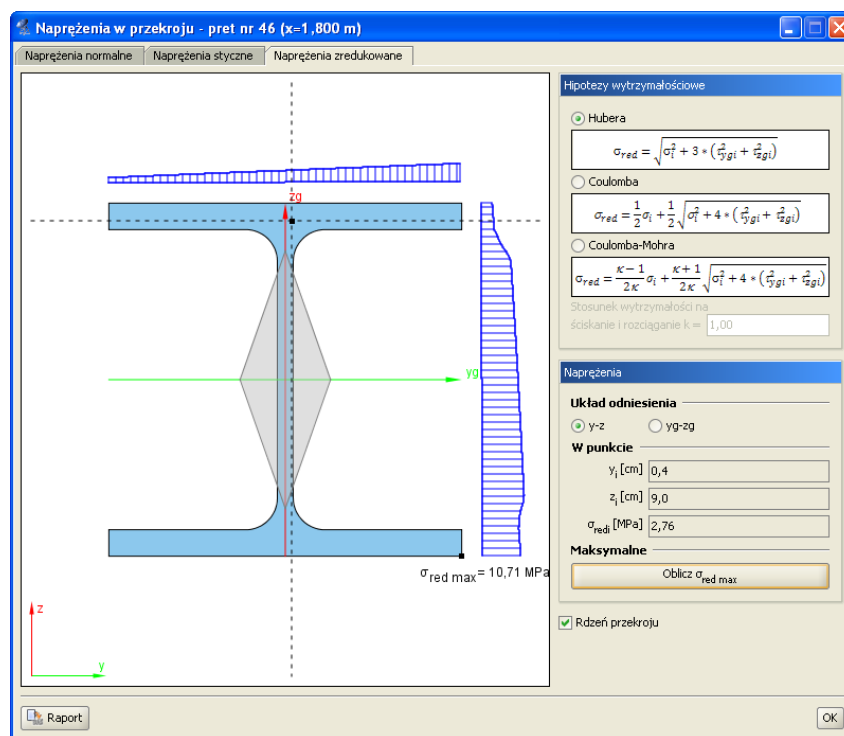
Rys. 3.70 Napężenia zredukowane w przekroju
