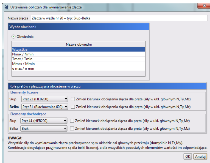
Okno definicji złącza Słup-Belka oraz Słup-Belka doczołowe
