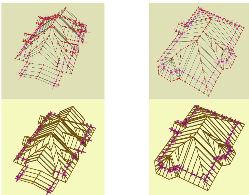
Rys. 2.19 Przykłady projektów dachów z systemu ArCADia z automatycznie wygenerowanym układem konstrukcji połaci w modelu siatkowym i widoku 3D
