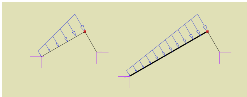
Rys. 3.62 Wydłużenie o podaną wartość pręta podpartego o końcu swobodnym
