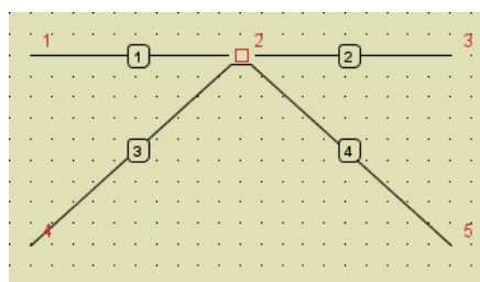
Pręty nr 3 i 4 zesztynwione, a nr 1 i 2 przegubowe
