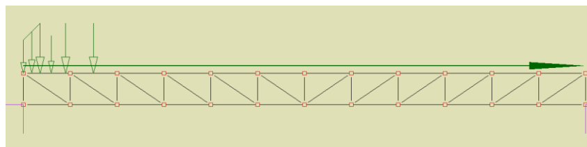
Rys. 7.18 Widok wprowadzonego obciążenia ruchomego
