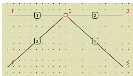
Pręty nr 1 i 2 zesztynwione, a nr 3 i 4 przegubowe
