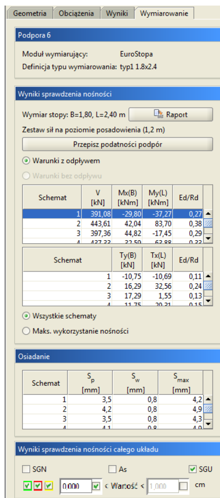
Rys. 14.25 Widok zakładki Wymiarowanie dla zaznaczonego węzła podporowego
