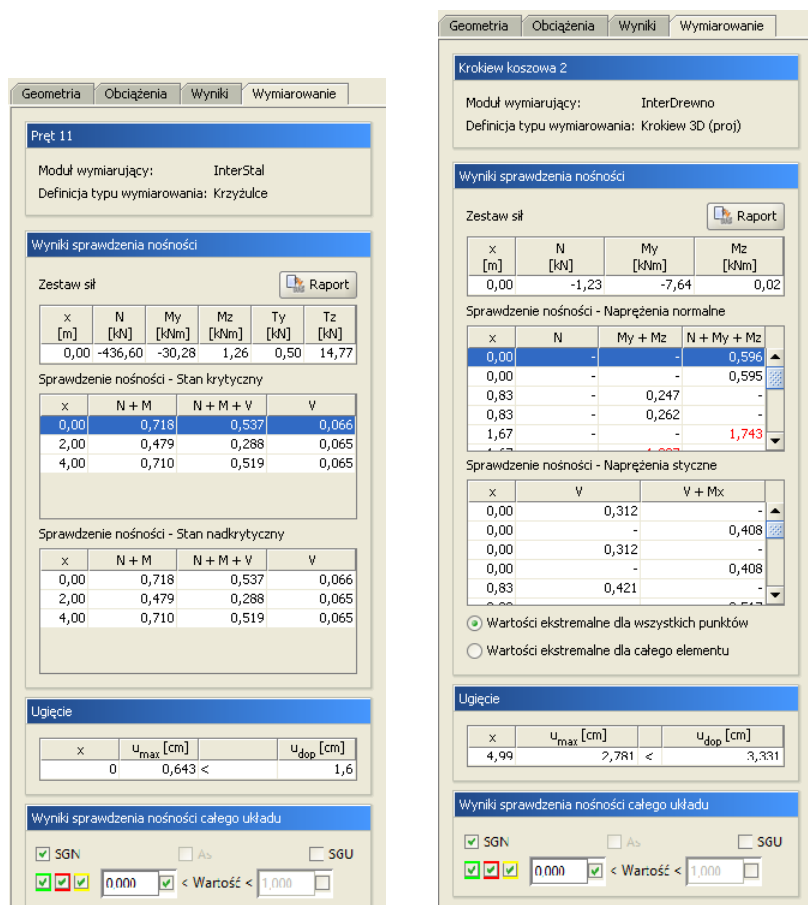
Rys. 14.17 Widok zakładki Wymiarowanie dla elementu drewnianego i stalowego według norm PN
