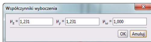
Okno edycji współczynników długości wyboczenia
