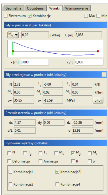
Rys. 3.14 Okno zakładki Wyniki przy zdefiniowanych kombinacjach
