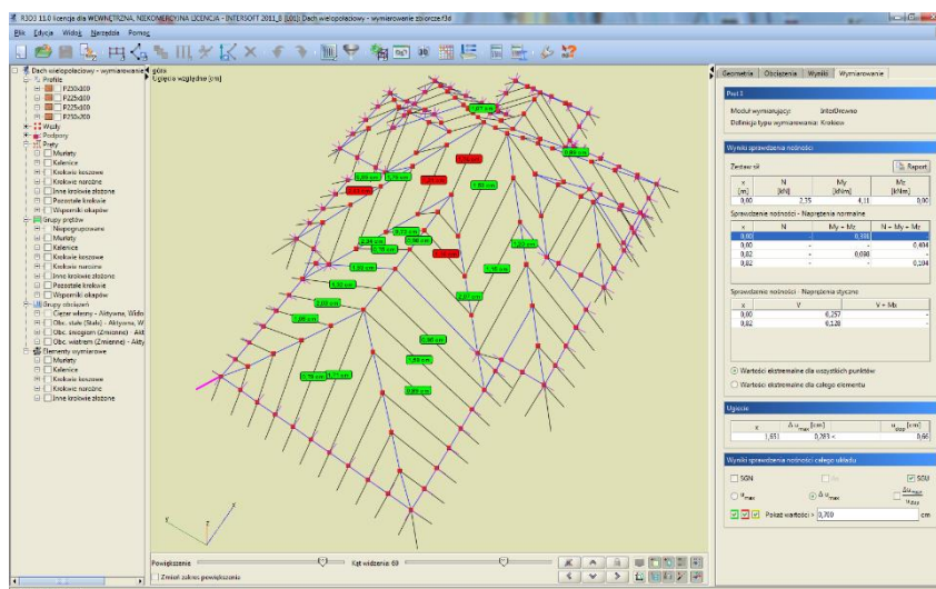
Rys. 14.23 Widok wyników wymiarowania zbiorczego dla stanu granicznego użytkownika
