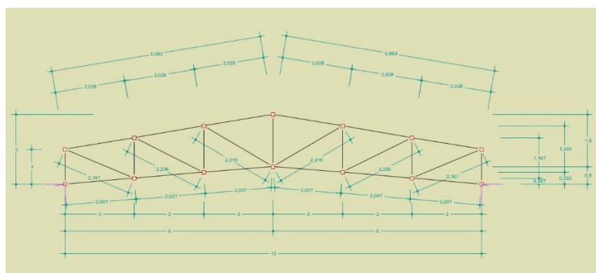
Rys. 3.15 Przykład projektu kratownicy z wstawionymi wymiarami
