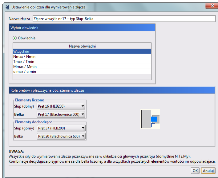
Okno definicji złącza Slup-Belka
