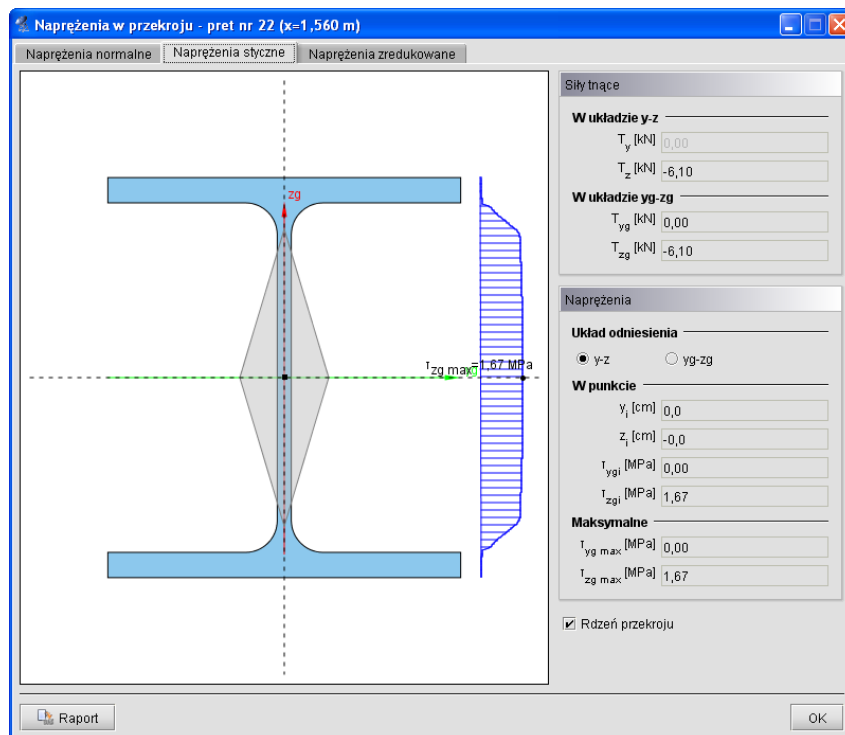
Rys. 3.61 Napężenia styczne w przekroju
