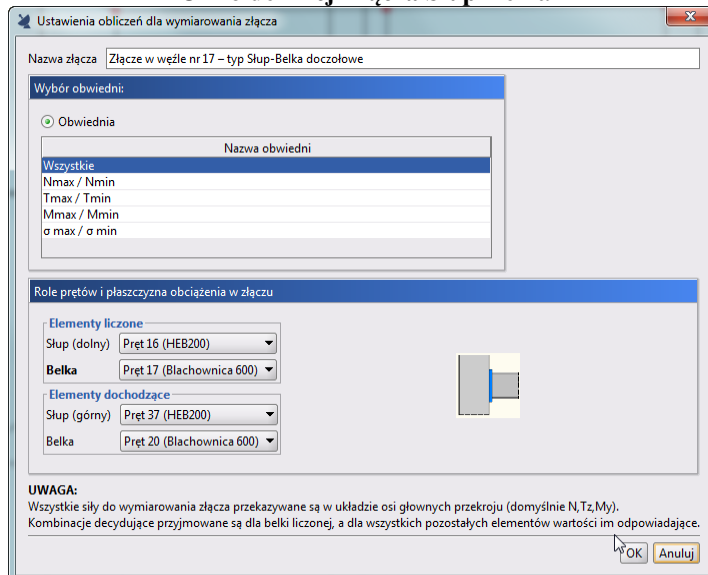
Okno definicji złącza Slup-Belka doczołowe
