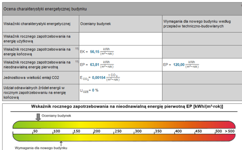
Fragment pierwszej strony świadectwa – metoda zużyciowa, wspólny system c.o. i c.w.u. Brak wartości wskaźnika EU
