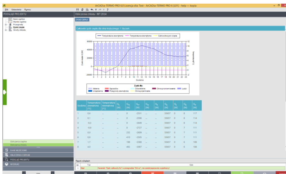
Raport Obliczenia chłodu - zyski ciepła
