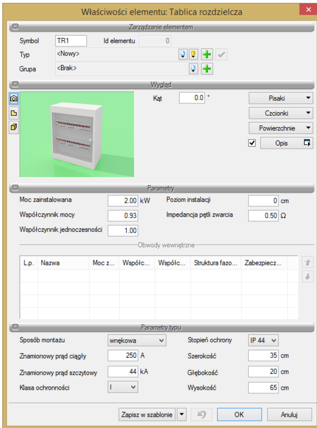
Rys. 11. Okno własności tablicy rozdzielczej
