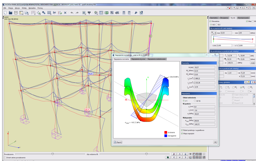
R3D3-Rama 3D: Gradientowe mapy naprężeń
